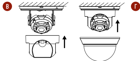
Рис. 2 Установка видеокамеры Н1Т ×0 на потолок
