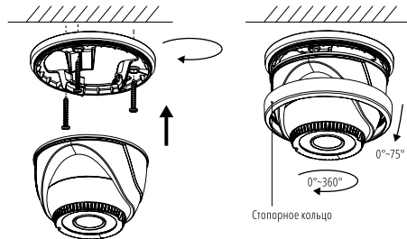
Рис. 8 Установка видеокамеры НІТ ×7
