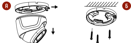
Рис. 3 Установка видеокамеры Н1Т ×2
