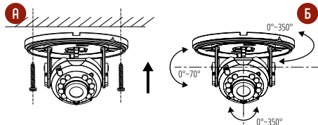
Рис. 1 Установка видеокамеры Н1Т ×0
