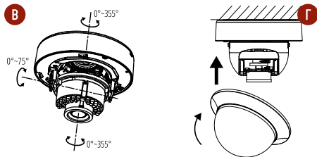
Рис. 7 Установка видеокамеры НІТ ×6
