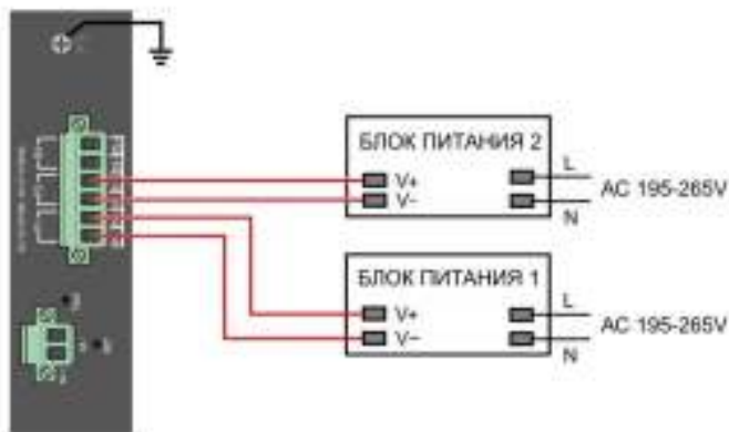
Рис.8 Схема подключения блоков питания к коммутаторам SW-80402/ILS(port 90W 180W) и SW-80802/ILS(port 90W 300W)
