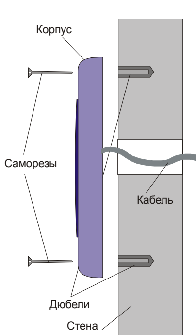
Рисунок 1. Крепление счетчика PR-P05. Рисунок 2. Крепление счетчика PR-P09.
