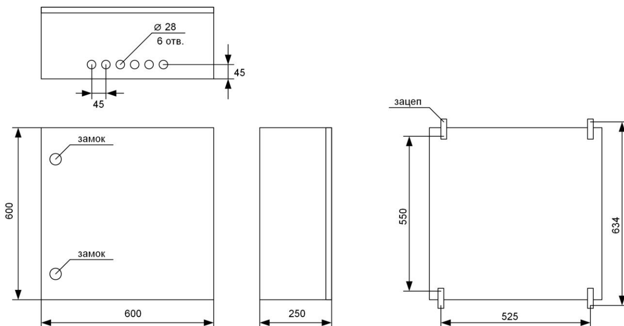
Рис. 8. Чертеж
