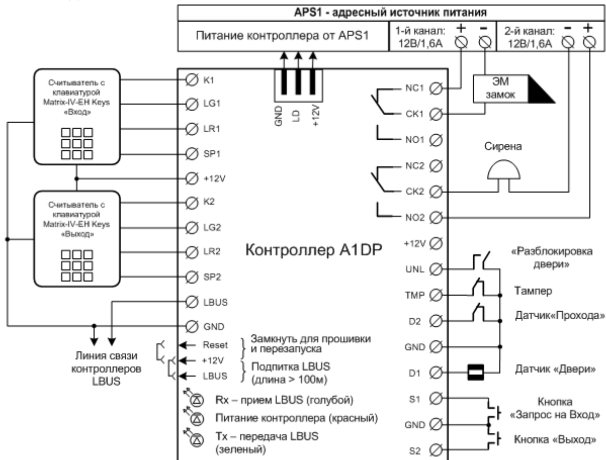
Рисунок 2 Схема подключения
