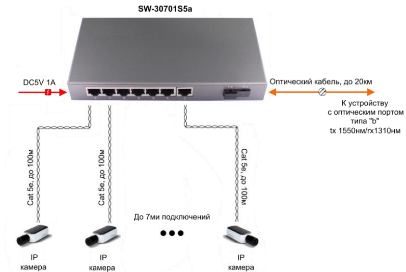
Рис. 11 Типовая схема подключения коммутатора SW-30701S5a
