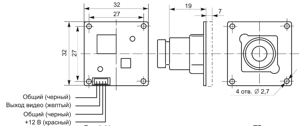
Рис.1. Установочные размеры и схема подключения ТВ камеры.
