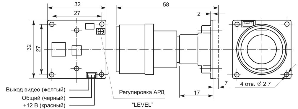
Рис.1. Установочные размеры и схема подключения ТВ камеры.
