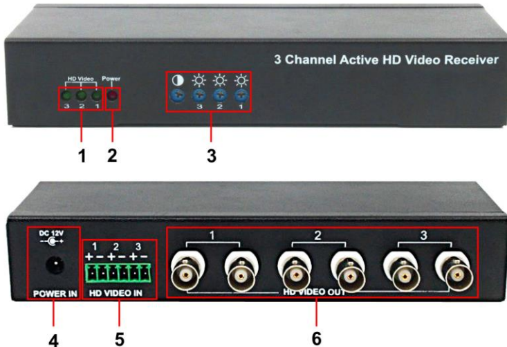
Рис. 2 Активный приемник RA-H3/2, разъемы, индикаторы и элементы регулировки на передней и задней панелях
