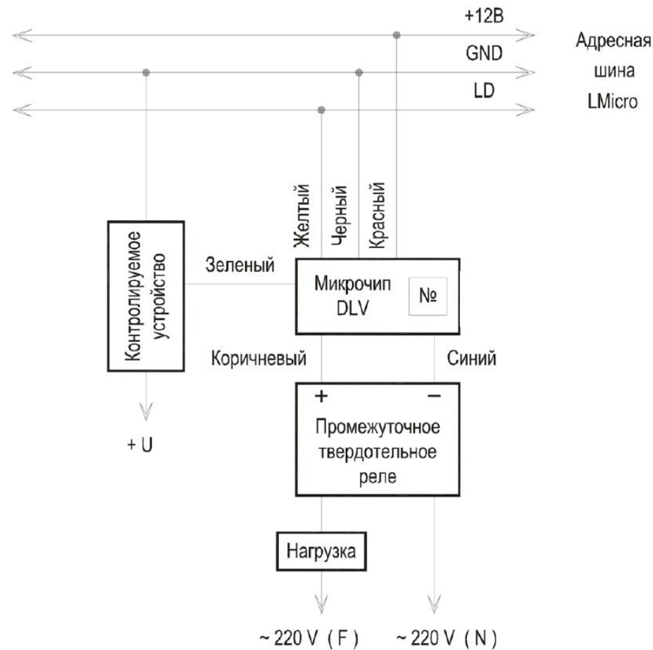
Рис.1. Схема подключения адресного микрочипа DLV
