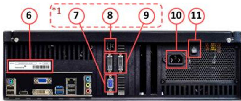
Рисунок 2. Задняя панель
