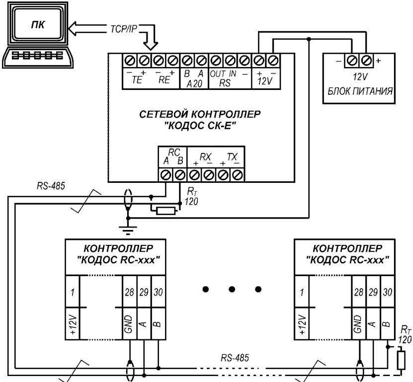
Рис. 4. Схема подключения к сетевому контроллеру "КОДОС СК-Е" контроллеров доступа серий "КОДОС RC", "КОДОС RCV"
