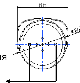
Вид сзади
