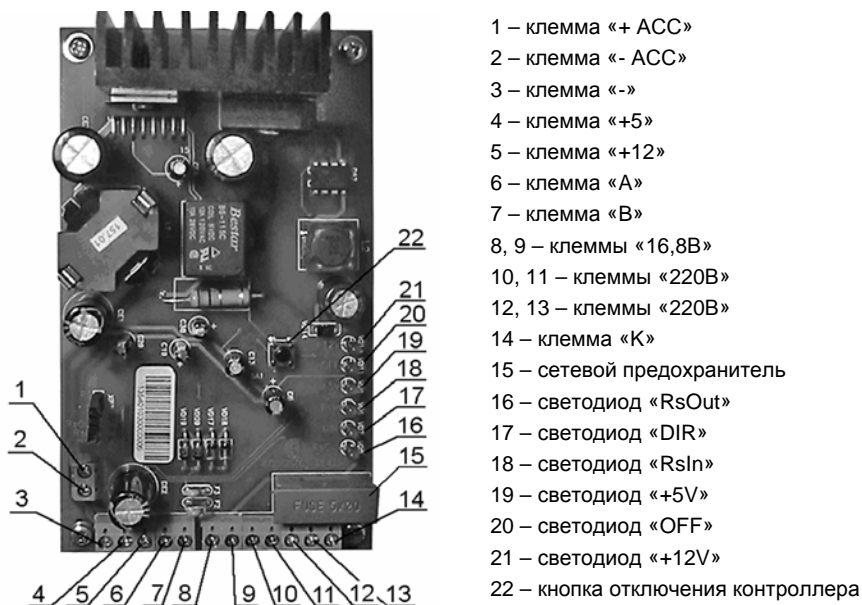
Рисунок 3 – Плата блока управления контроллера
