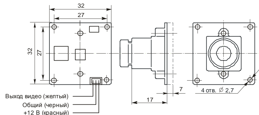
Рис.1. Установочные размеры и схема подключения ТВ камеры.
