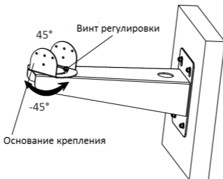
Рисунок 2-4 Регулировка угла наблюдения
