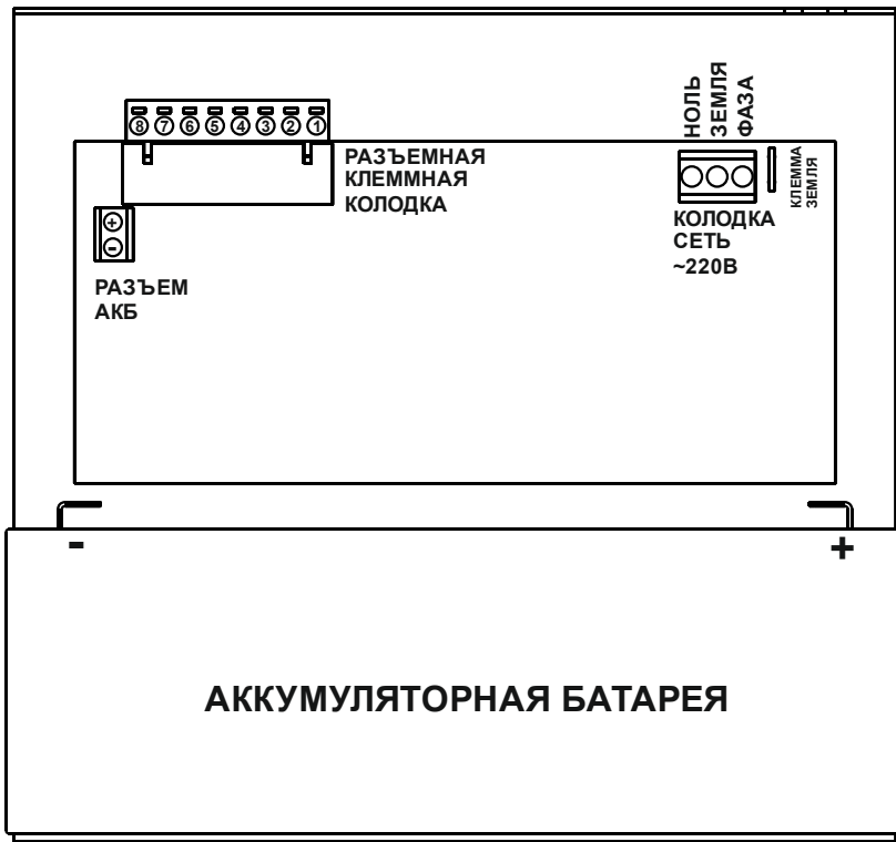
РИСУНОК 3 – Вид источника с нижней стороны без днища.
