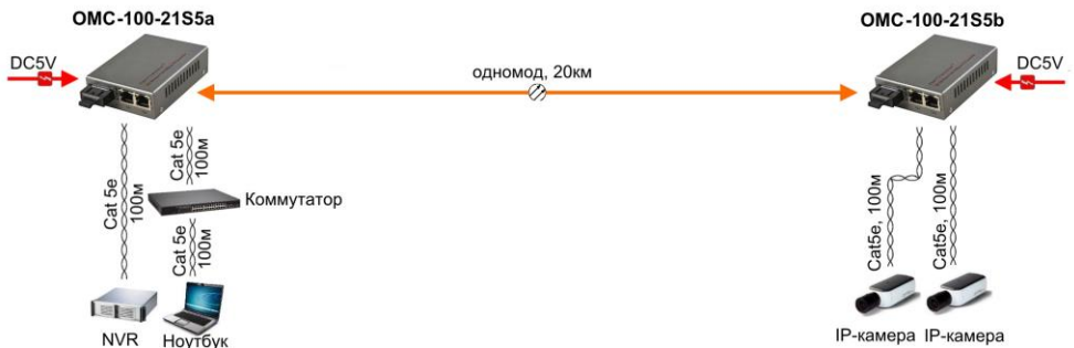
Рис. 7 Схема подключения медиаконвертеров OMC-100-21S5a (OMC-100-21S5b)
