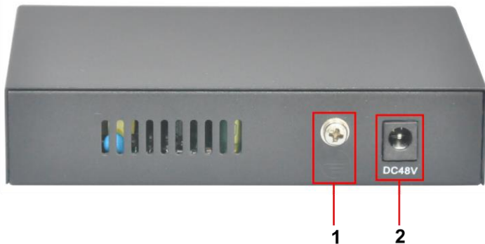
Рис. 3 Коммутатор SW-20500/B(ver.2), разъемы и клеммы на задней панели
