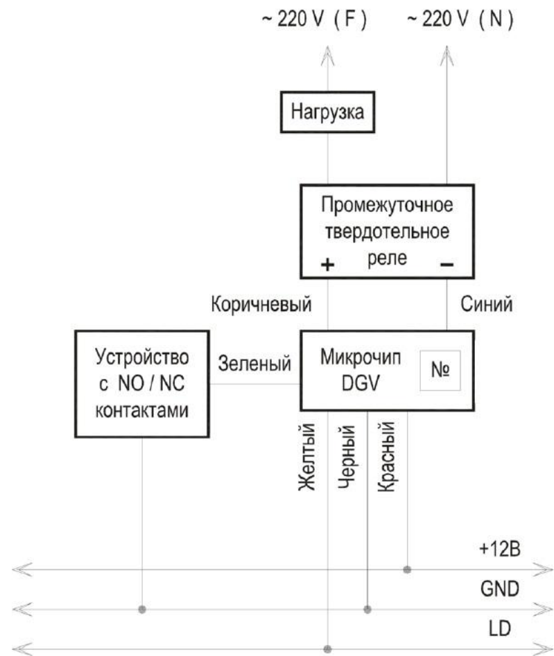
Рис.1. Схема подключения адресного микрочипа DGV
