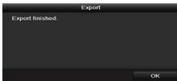
Рисунок 7.34 Экспорт завершен
