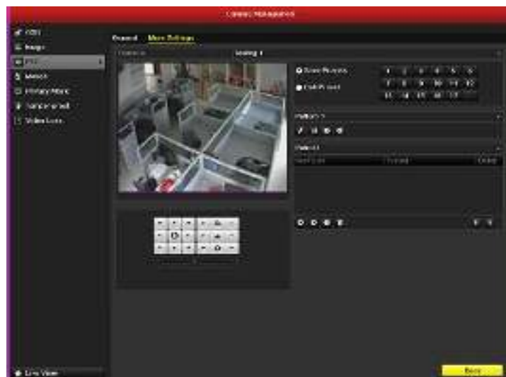
Рис 4.11 PTZ- шаблоны
