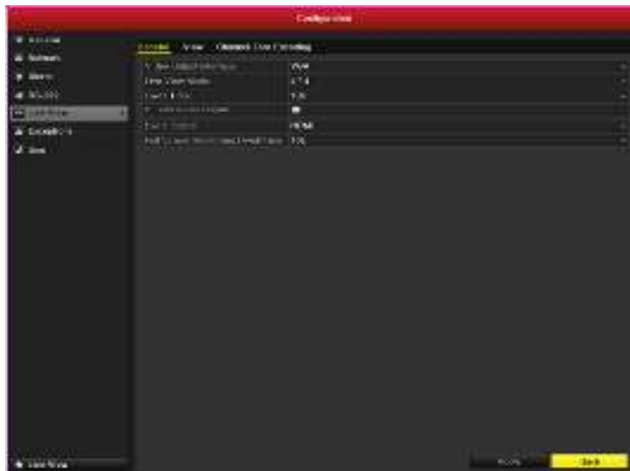
Рис. 3.6 Отображение - Основные
