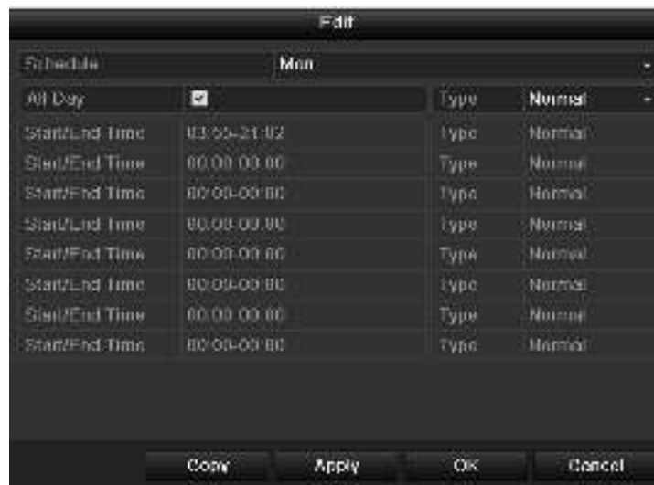
Рис 5.8 Редактирование расписания
