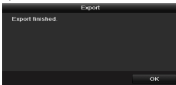
Рисунок 7.13 Экспорт завершен
