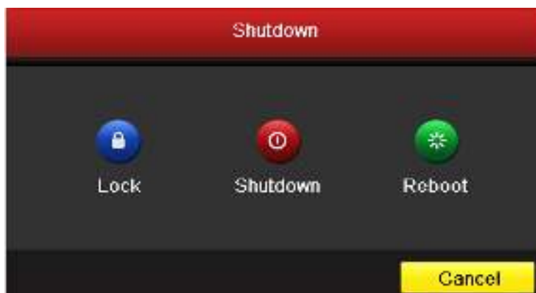
Рисунок 1.9 Меню выключения
