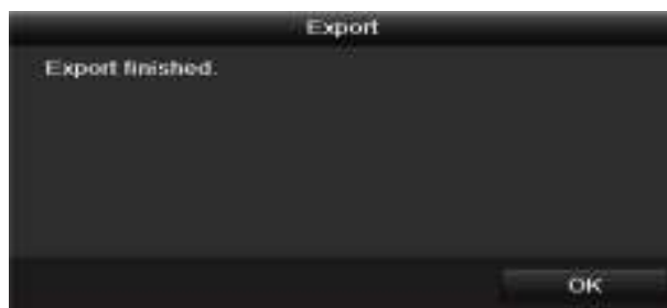
Рисунок 7.18 Экспорт завершен
