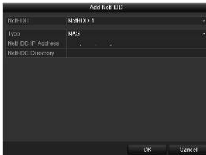
Рисунок 10.6 Добавление NetHDD
