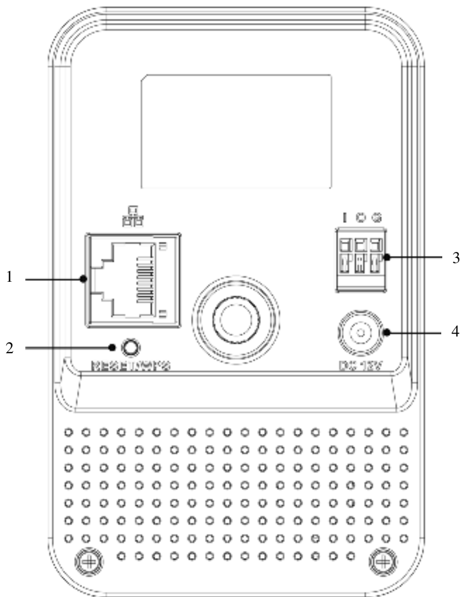
Рис. 1 Разъемы видеокамеры
