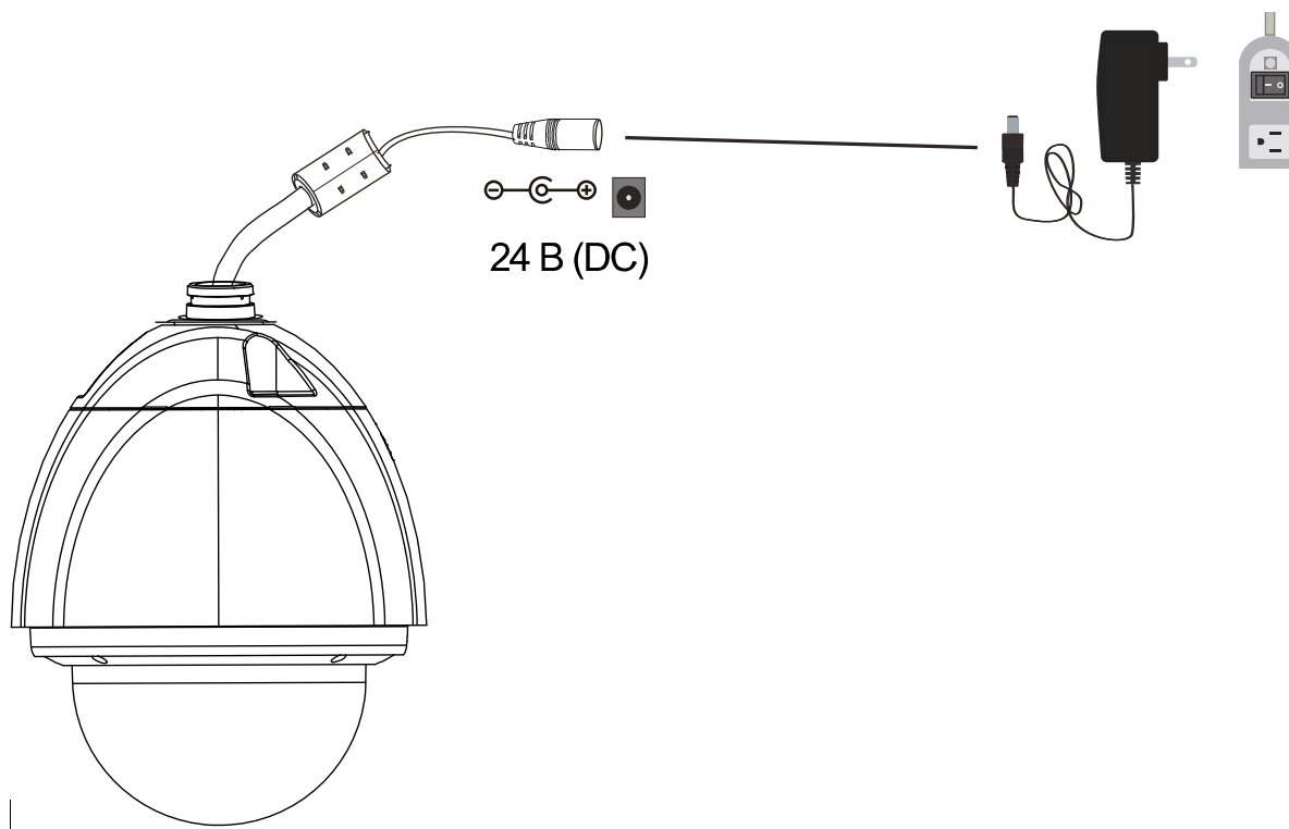
Рис. 4.3.1.1. Контакты питания
