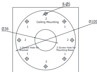
Рисунок 2-10 Сверление отверстий в стене
