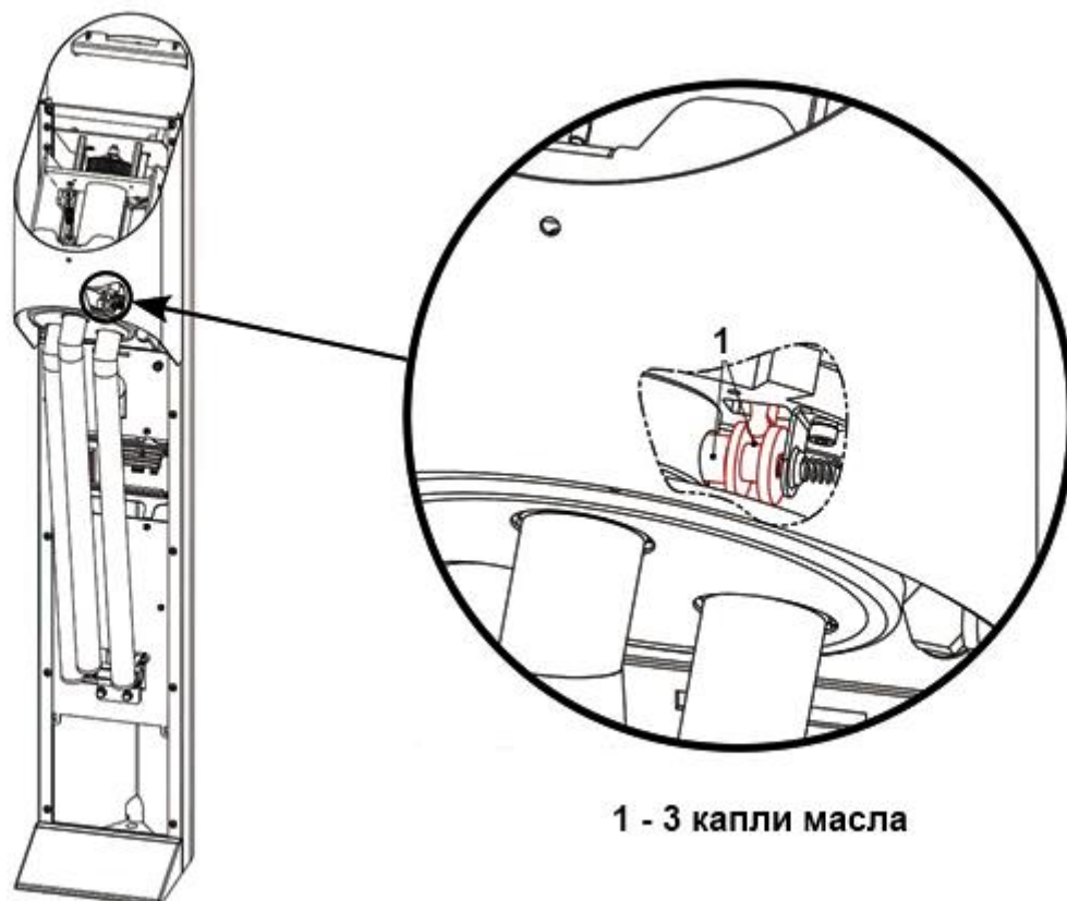
Рисунок 26 – Места соединения фиксатора и кулачка разблокировки планок (центральная стойка турникета)
