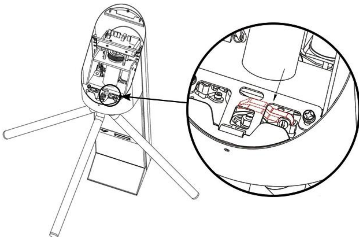
Рисунок 16 – Сложение планок турникета (центральная стойка турникета)
