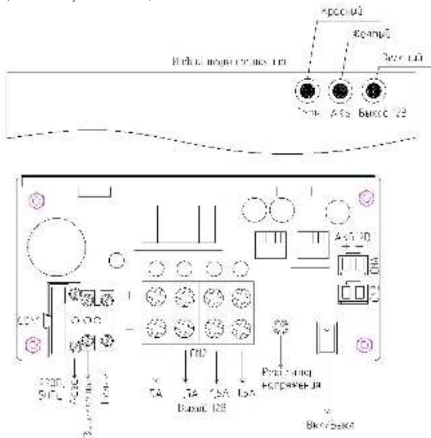
Рисунок 1 Схема подключения Optimus 1250-09-12
