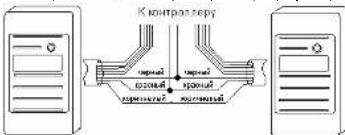
Рисунок 3 – Подключение синхронизированных считывателей
