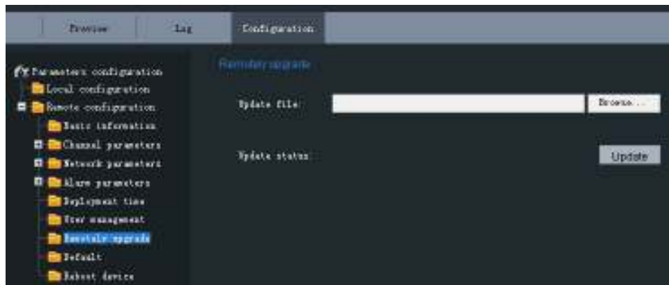
Рисунок 2.1.28: Удаленное обновление.
