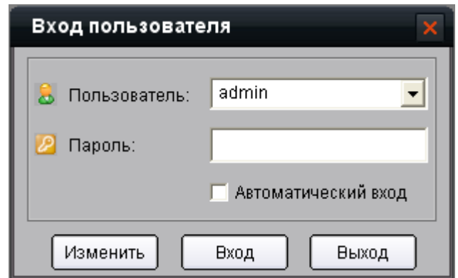
Рисунок 2.12: Вход пользователя.
