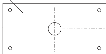
МОНТАЖНОЕ ОСНОВАНИЕ ТУМБЫ ШЛАГБАУМА
