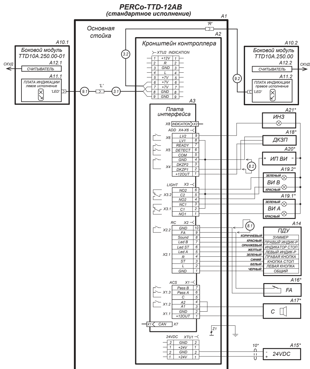
Схема подключения турникета TTD-12AB
