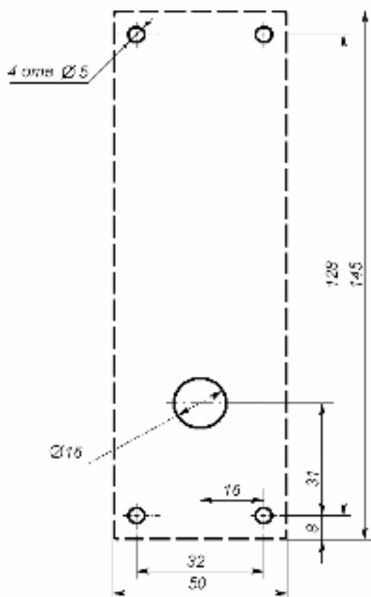
Рисунок 3 Разметка отверстий для установки считывателя (пунктиром показаны габариты корпуса считывателя)
