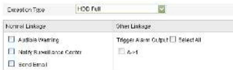
Рисунок 6-33 Настройки исключений
