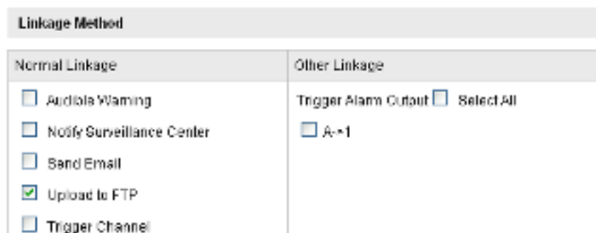
Рисунок 6-28 Методы связи
