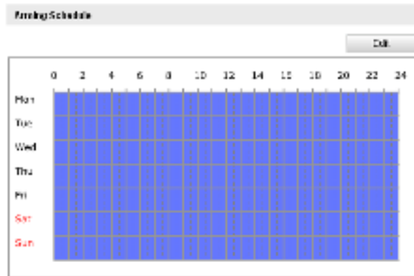
Рисунок 6-26 Время активности
