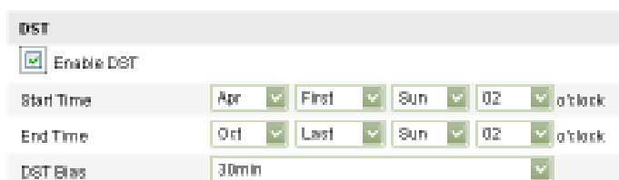
Рисунок 6-6 Настройки DST
