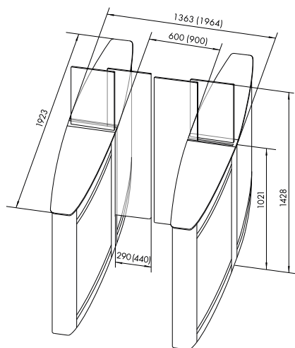
Габаритные размеры
