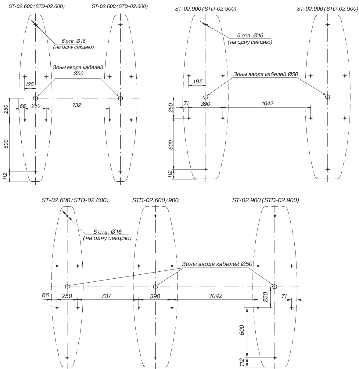
Разметка отверстий в полу под крепление стойки турникета и зона для подводки кабелей
