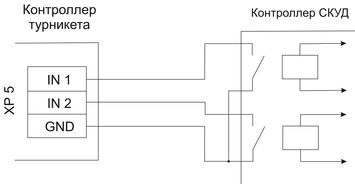
Рисунок 8.2.2 Подключение турникета к стороннему СКУД
