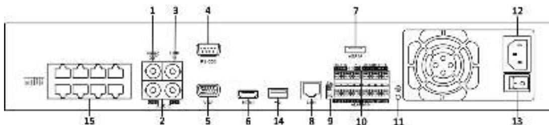
Рис. 1.11 DS-7708NI-SP
