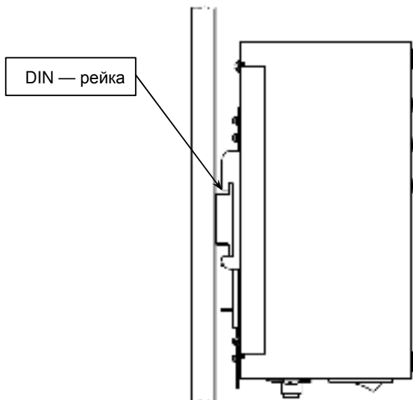
Рисунок 4 – установка изделия на DIN-рейку
