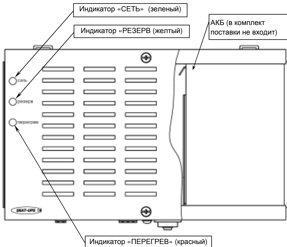
Рисунок 1 - общий вид изделия с установленной АКБ
