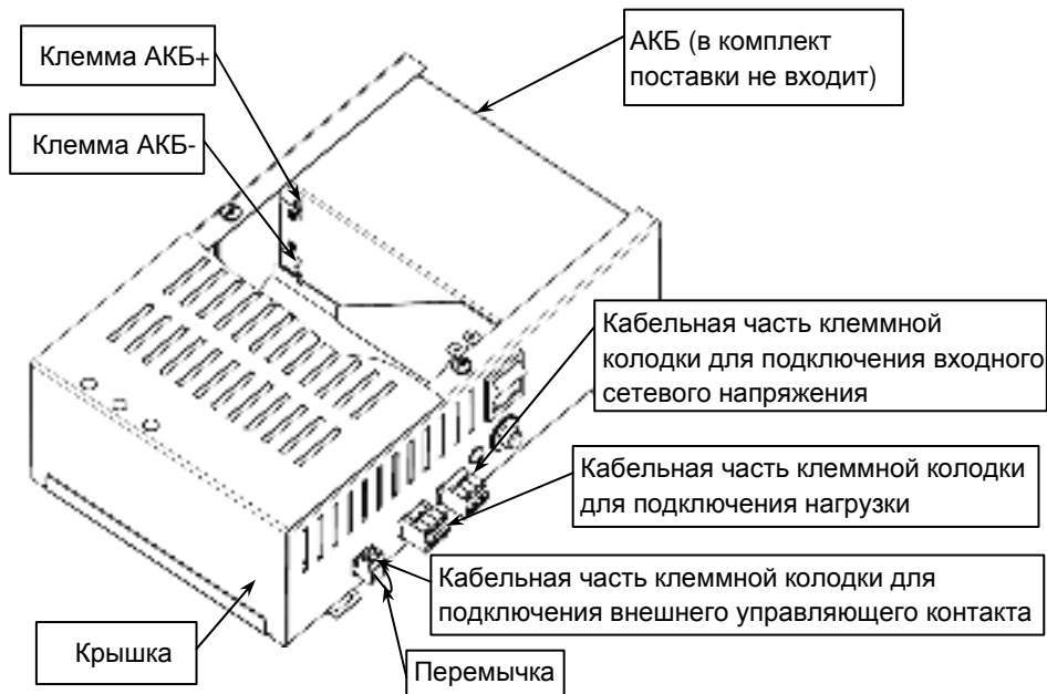
Рисунок 3 — расположение АКБ и кабельных частей колодок
