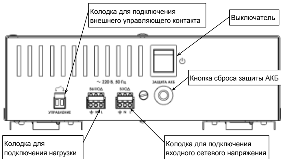
Рисунок 2- вид изделия со стороны подключения
