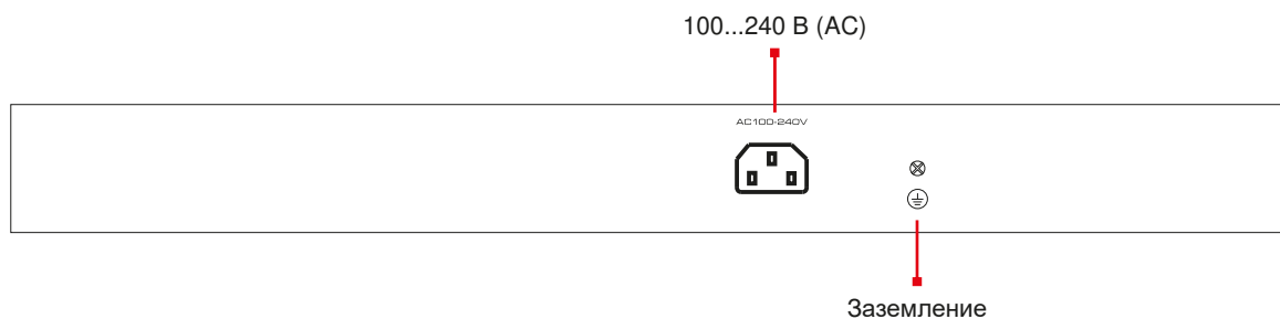
Рис. 2.3. Задняя панель
