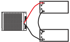
Схема подключения 2-х АКБ 12В
