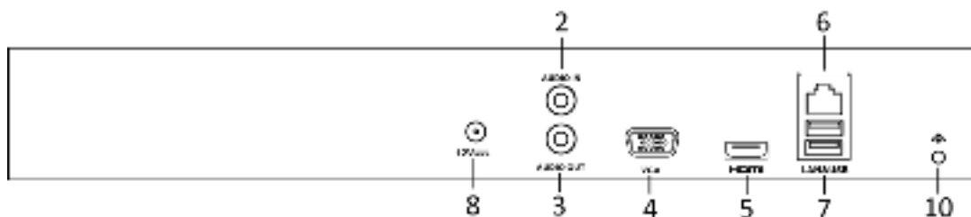
Рисунок 1-14 Серия DS-7600NI-K1
