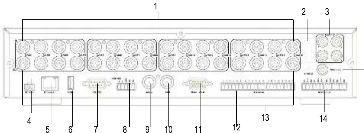
Рисунок 1-2 Задняя панель
