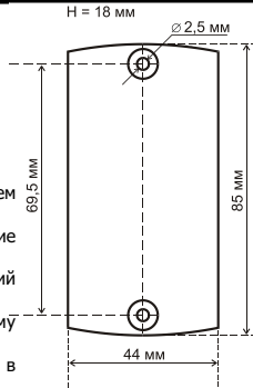
Рис.2 Габаритные размеры
