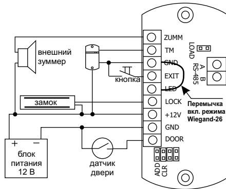
Рис.3 Подключение устройств
