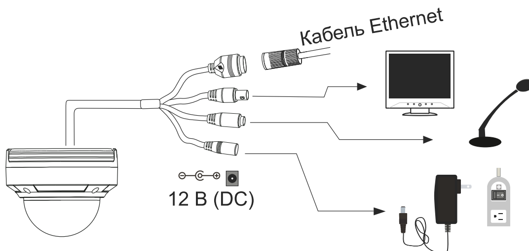
Рис. 3.2. Подключение кабелей
