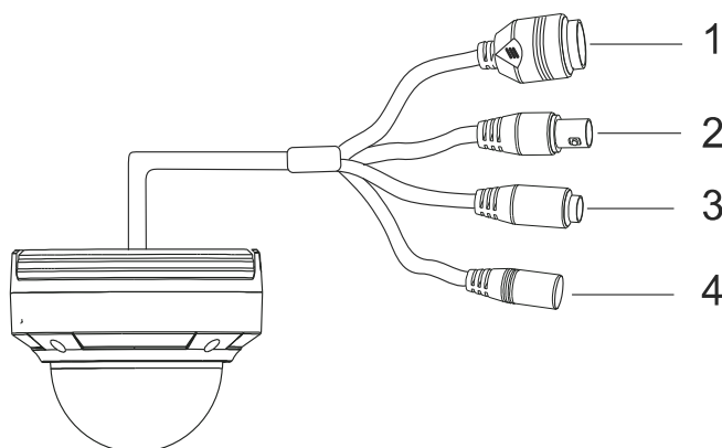
Рис. 3.1. Внешний вид
