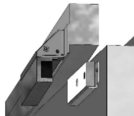
Рисунок 4 - Установка замка с монтажным комплектом МК AL-350FB-M-01
