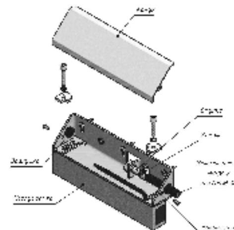
Рисунок 11 – Крепление корпуса замка с помощью комплекта МК AL-350FB-M-02 для прокладки кабеля в металлорукаве
