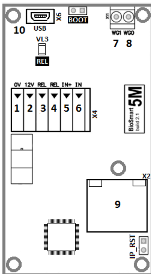
Внешний вид платы контроллера
