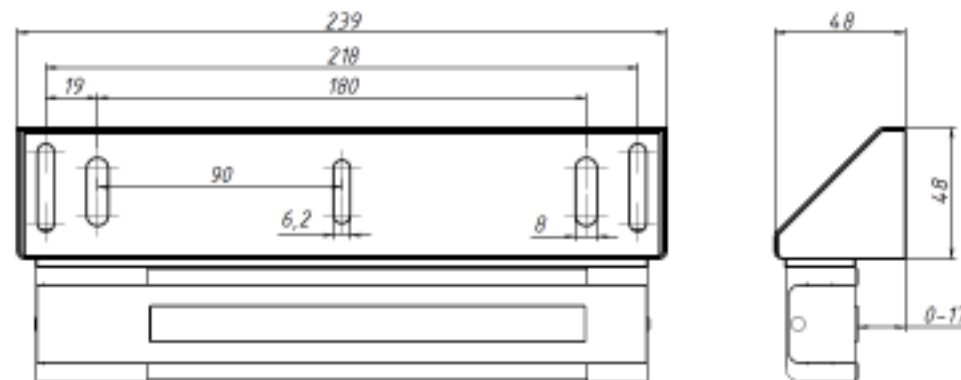
Рисунок 2 – Габаритный чертеж
