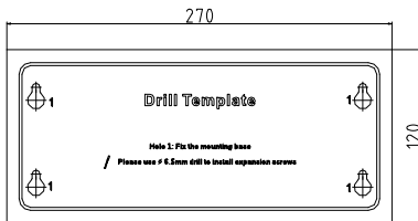
Рисунок 2-7 Шаблон крепления
