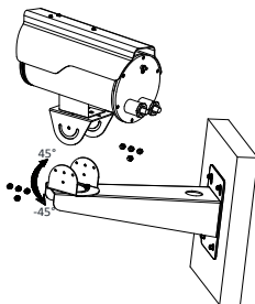
Рисунок 2-5 Установка камеры на кронштейн
