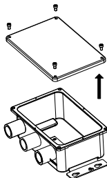
Рисунок 2-8 Демонтаж монтажной коробки
