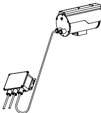
Рисунок 2-12 Установка крышки монтажной коробки
