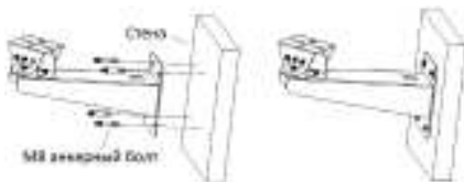
Рисунок 2-1 Установка кронштейна
