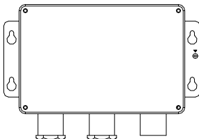
Рисунок 2-9 Установка монтажной коробки
