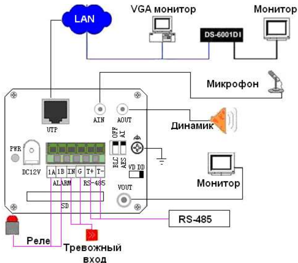
Рис. 2.3.1 Топологическая схема сетевой камеры серий DS-2CD792PF-E
