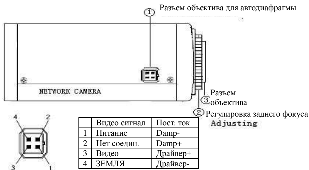
Рис. 2.2.1 Камеры серий DS-2CD792PF-E , DS-2CD832F-E– вид сбоку
