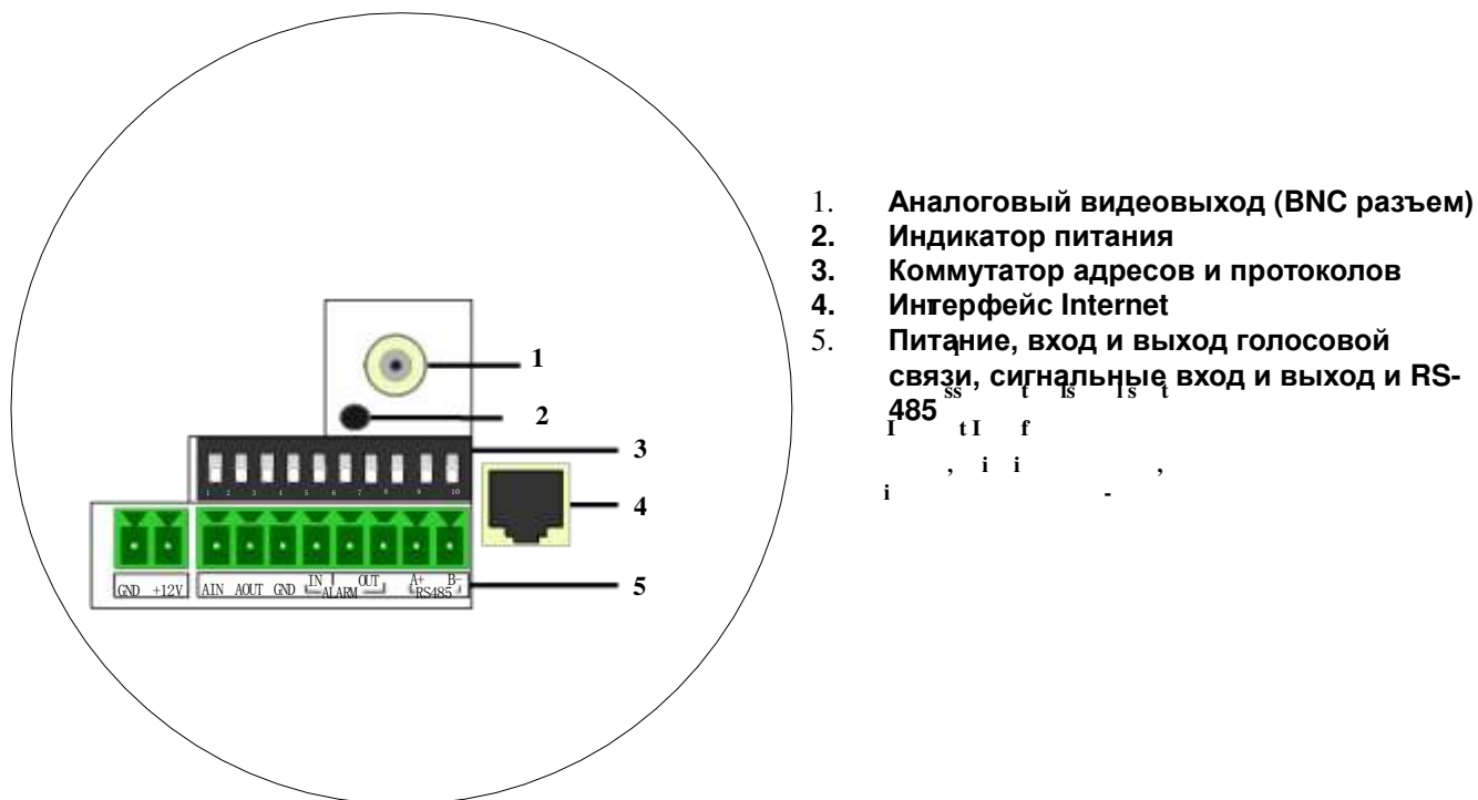
Рис. 2.2.7 Задняя панель камер серий: DS-2CD792PF-E, DS-2CD752MF-FB.
