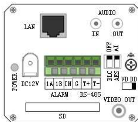
Рис. 2.2.5 Задняя панель серий DS-2CD792PF-E
