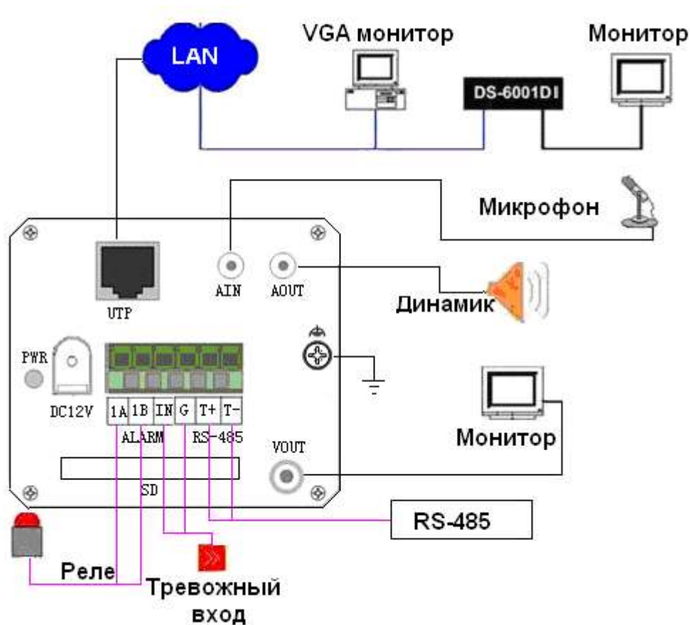
Рис. 2.3.1 Топологическая схема сетевой камеры серий DS-2CD832F-E, DS-2CD862MF-E, DS-2CD852MF-E
