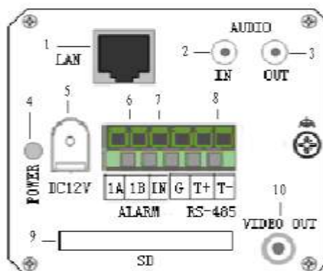
Рис. 2.2.4 Задняя панель серий BestIPcam-D300CMOS, DS-2CD852MF-E
