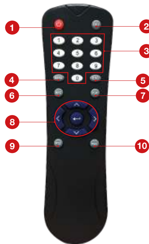
Рисунок 3.17 ИК пульт управления.
