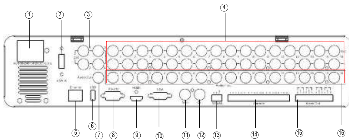
Рисунок 1-2 Задняя Панель
