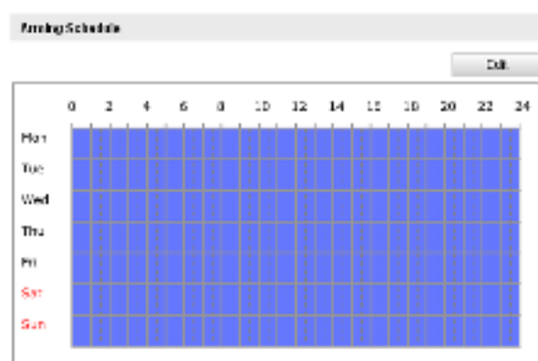
Рисунок 6-41 Время активности
