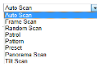
Рисунок 5-8 Тип действия
